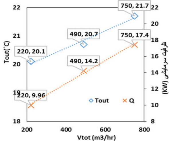
شکل (۱۳): ظرفیت سرمایش مخصوص و دمای خروجی کولر برحسب دمای ورودی برای سه دبی حجمی ورودی
