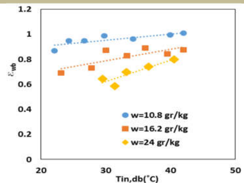
شکل (۹): بازده حباب مرطوب کولر بر حسب دمای ورودی
