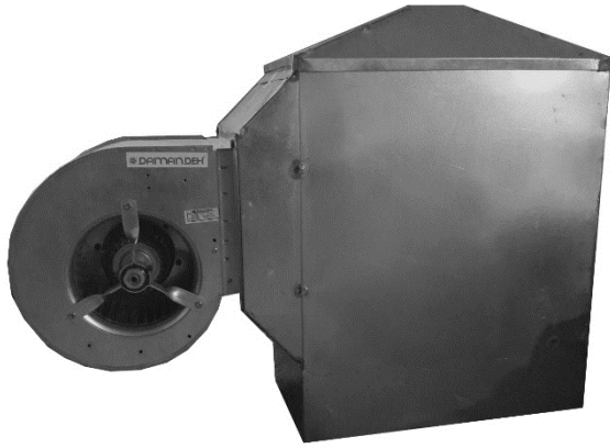
شکل (۲): کولر تبخیری غیرمستقیم با مبدل جریان عمود
