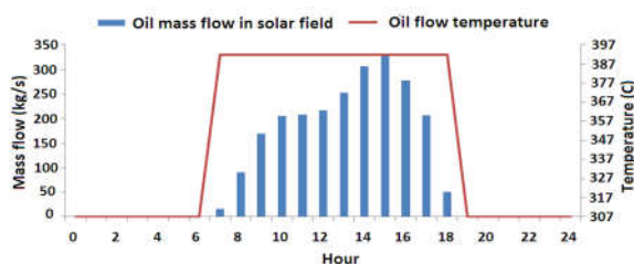
شکل (۷): نرخ جریان روغن و دمای خروجی روغن از میدان خورشیدی در روز طراحی
