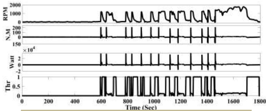
شکل (۱۱): عملکرد موتور احتراقی در سیکل رانندگی تهران با کنترل کننده فازی متداول
