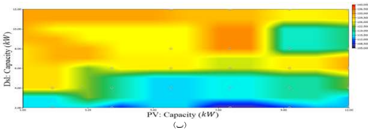
شکل (۱۱): اثر قیمت دیزل روی سیستم در حالت (الف) قیمت دیزل 0.16 \$/lit و در حالت (ب) قیمت دیزل 1/5 \$/lit
