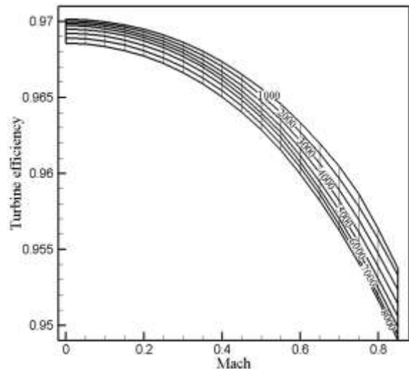
شکل (۱۰): نمودار تغییرات بازده انرژی توربین برحسب تغییرات ارتفاع و تغییرات عدد ماخ پروازی
