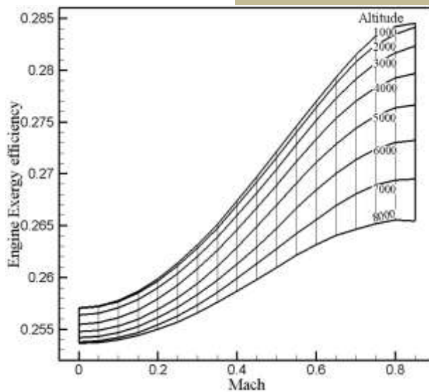
شکل (۱۲): نمودار تغییرات بازده انرژی موتور برحسب تغییرات ارتفاع و تغییرات عدد ماخ پروازی
