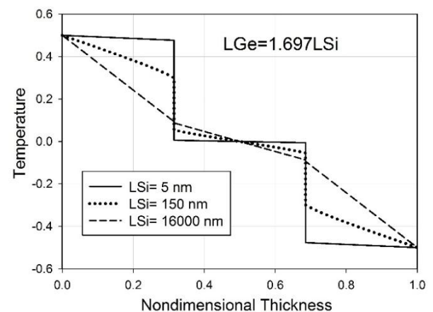
شکل (۹): پروفایل دما در عرض ابرشبهه (درصد اتمی ژرمانیوم ۶۰٪)
