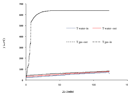
شکل (۹): تغییرات دمایی گاز ورودی و خروجی از آگزوز و آب ورودی و خروجی از مبدل حرارتی در بار ۷۵٪ موتور
