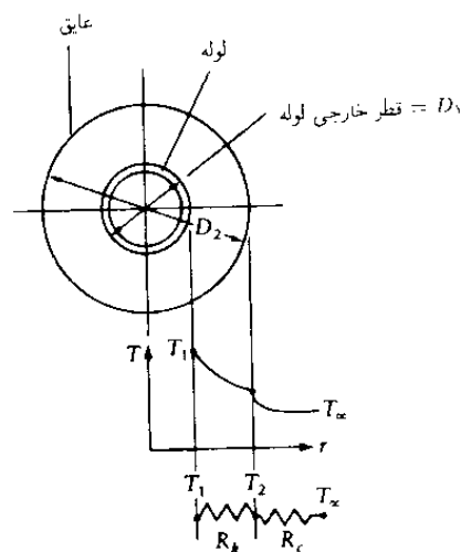
شکل (۲): لوله عایق دار
