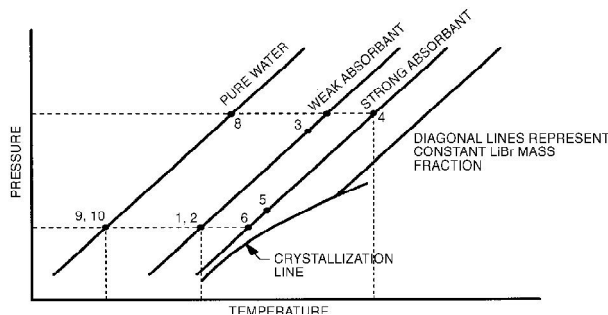
شکل (۲): نمودار دو خاصیتی لیتیم بروماید - آب [۷]
