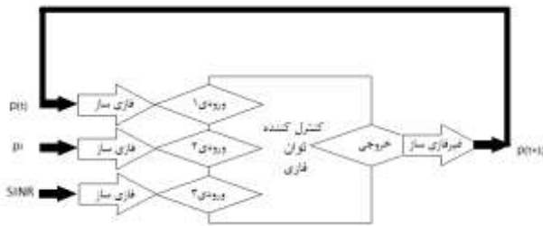
شکل (۳): نمای بیرونی کنترل‌کننده توان فازی
