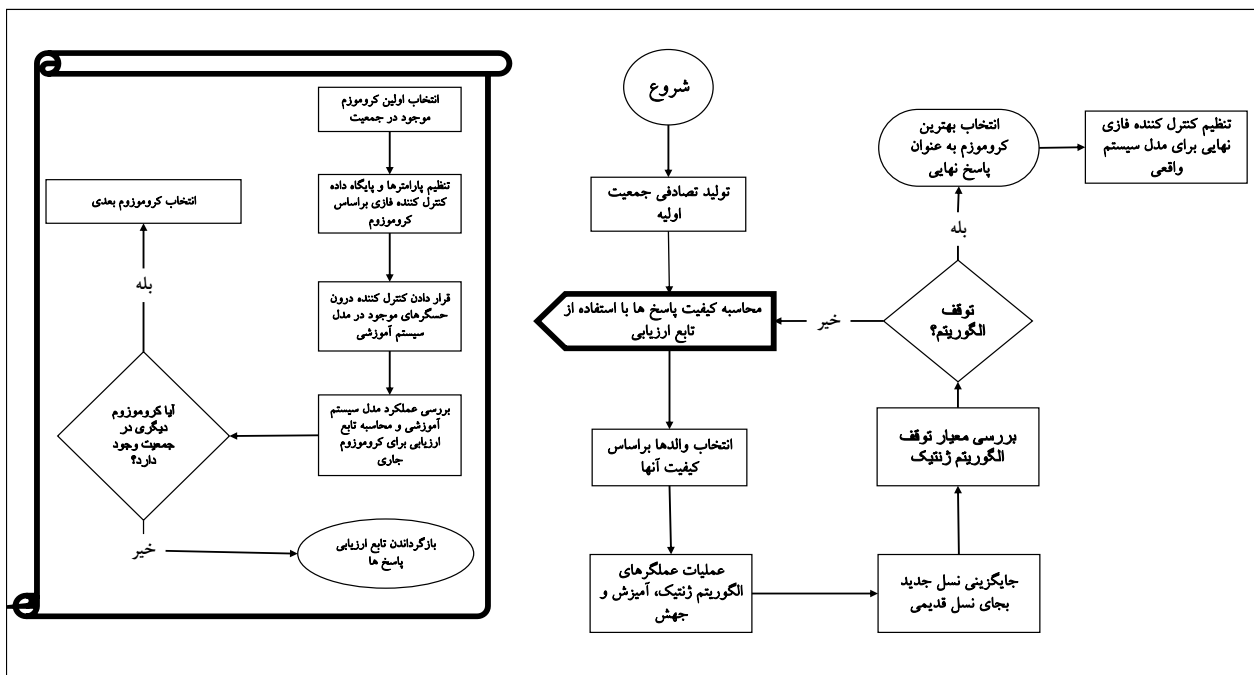
شکل (۶): روند نمای کلی الگوریتم ژنتیک فازی
