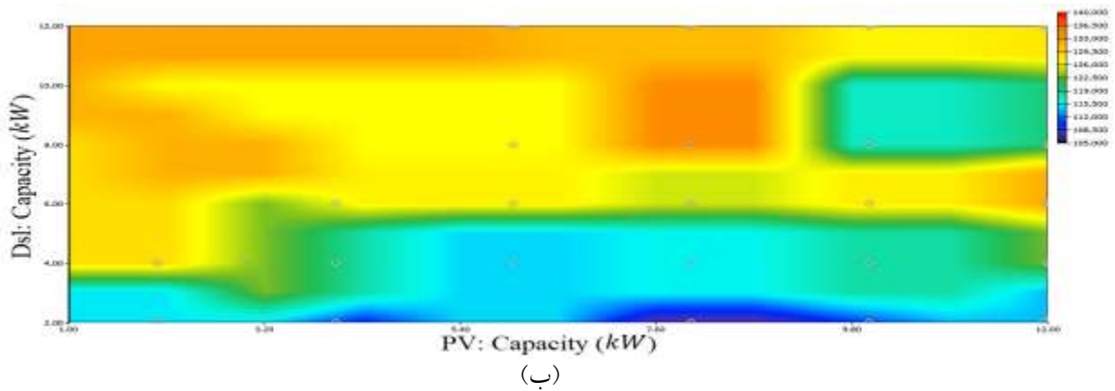
شکل (۱۱): اثر قیمت دیزل روی سیستم در حالت (الف) قیمت دیزل 0.06 \$/lit و در حالت (ب) قیمت دیزل 0.15 \$/lit
