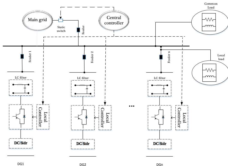
شکل (۱): ساختار یک ریزشبه نمونه با حضور n ریزمنبع
