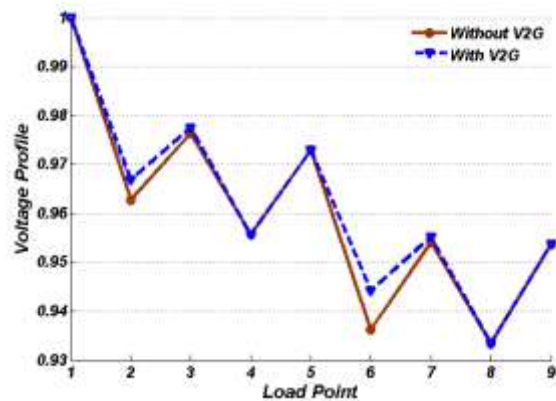
شکل (۸): پروفیل ولتاژ در یک ساعت پرباری و یک ساعت کم‌باری
