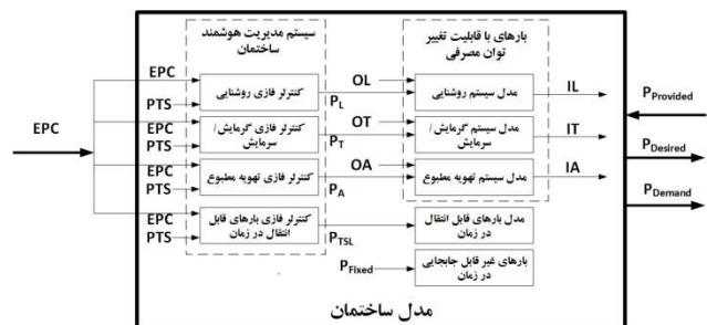
شکل (۱): بلوک دیاگرام ساختمان هوشمند
