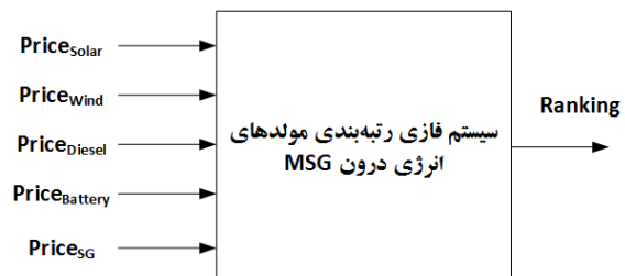
شکل (۲): سیستم فازی رتبه‌بندی مولدهای انرژی درون MSG
