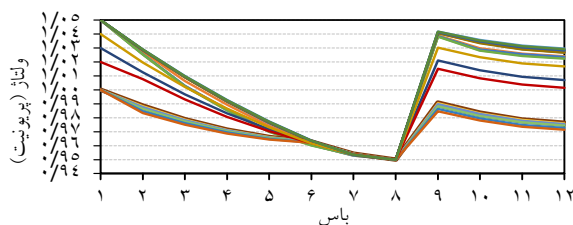
شکل (۵): منحنی ولتاژ گره‌ها در ۲۴ ساعت (سناریوی ۱)
