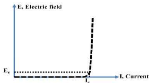
شکل (۲): مشخصه ولتاژ-جریان HTS
