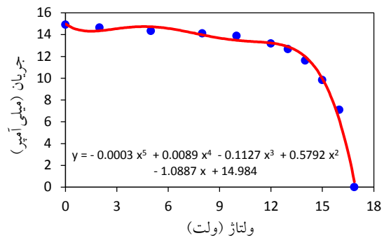
شکل (۴): نمونه‌ای از منحنی برازش شده بر داده‌های جریان-ولتاژ
