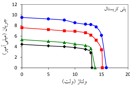
شکل (۵): منحنی مشخصه جریان-ولتاژ (I-V) در سطوح مختلف
