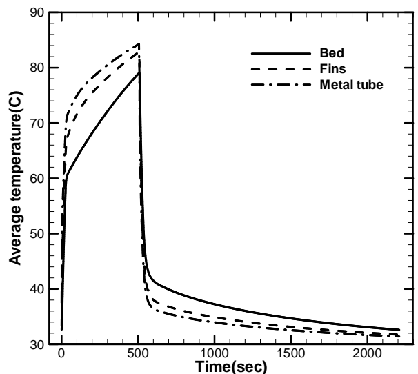
شکل (5): تغییرات دمای میانگین لوله فلزی، پرها و بستر ماده جاذب
