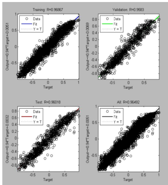
شکل (۲): نتایج الگوریتم لونیگ-مارکات در برنامه متلب
