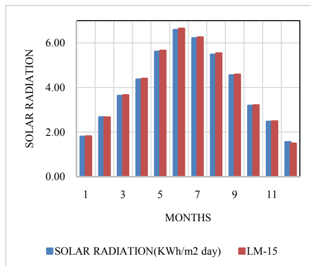
شکل (۳): مقایسه داده‌های هواشناسی ایستگاه تبریز و الگوریتم LM در ۱۲ ماه سال
