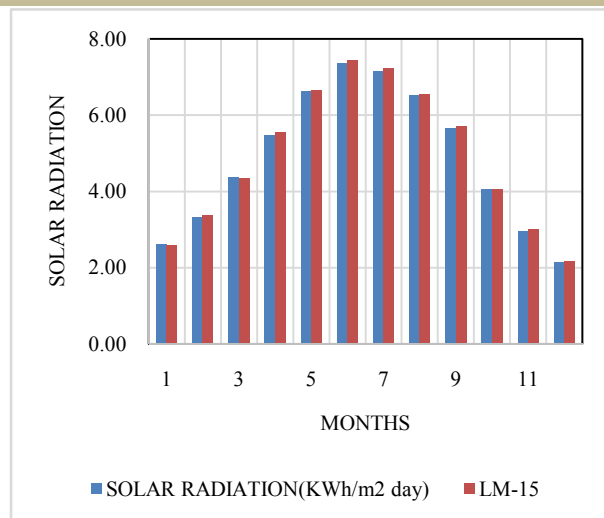
شکل (۴): مقایسه داده‌های هواشناسی ایستگاه تهران و الگوریتم LM در ۱۲ ماه سال
