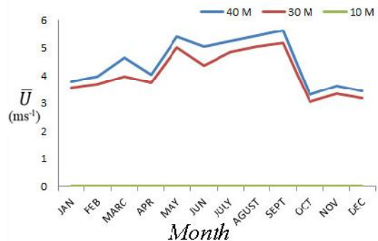
شکل (4): سرعت متوسط ماهانه باد در دهک [15]
