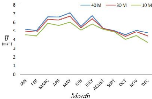
شکل (2): سرعت متوسط ماهانه باد در چابهار [15]
