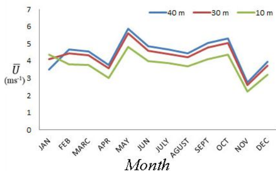
شکل (3): سرعت متوسط ماهانه باد در دلگان [15]
